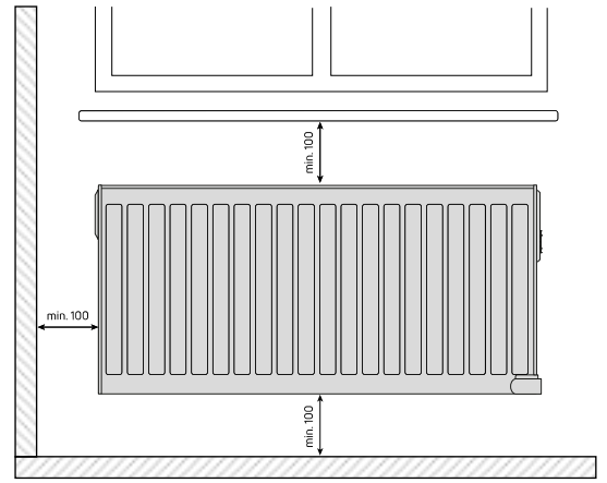
Minimivstånd vid installation
