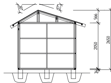
Sektion
