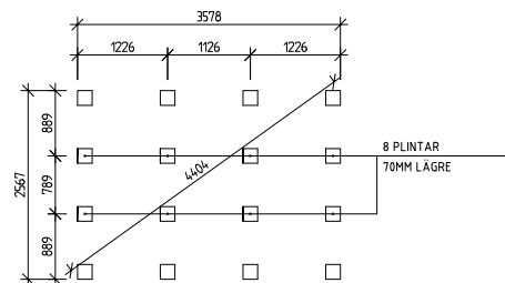
Plintritning
