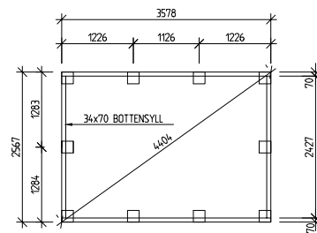
Sektion
