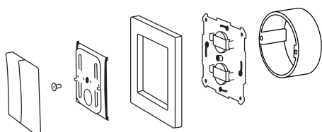
Montage utanpå apparatdosa med skruv.
