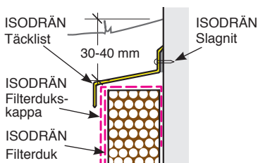
Detalj: Montering ISODRÄN Filterdukskappa.
