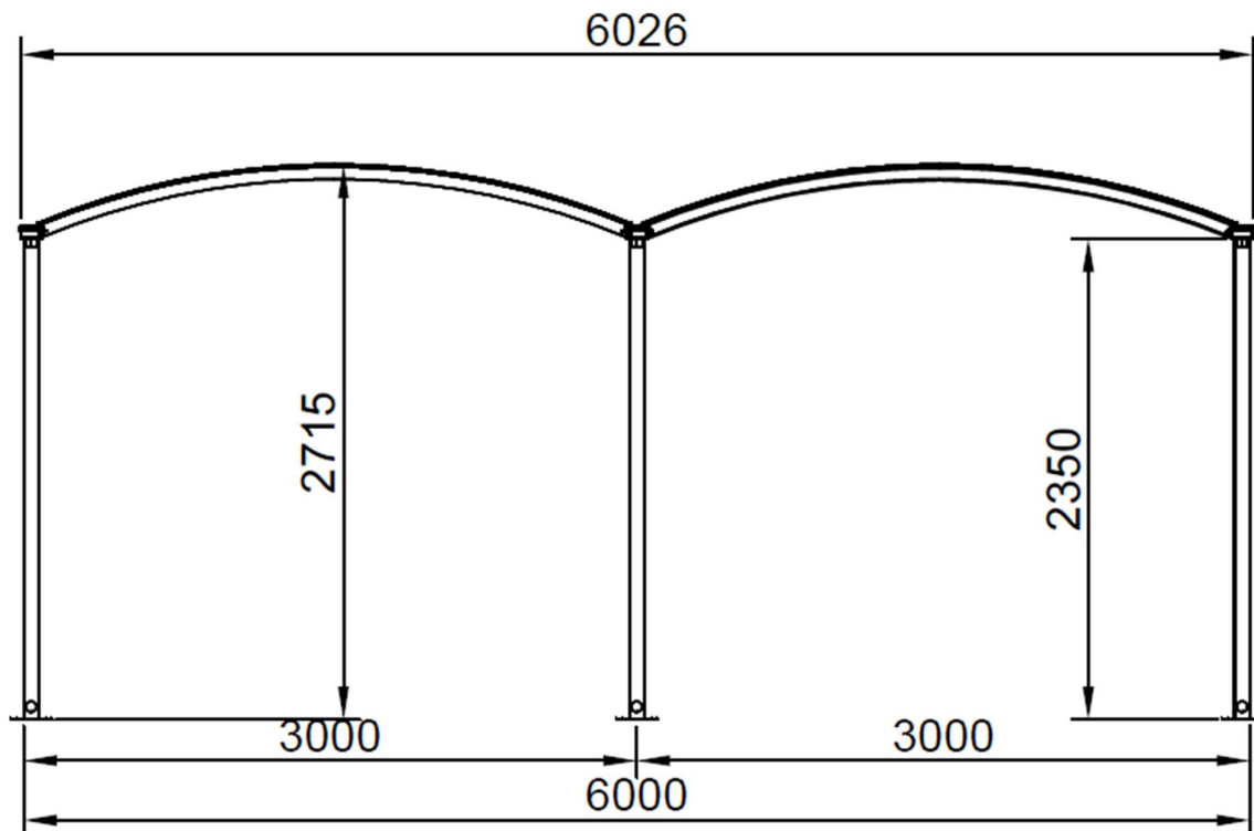
Mål tegning (set forfra)
