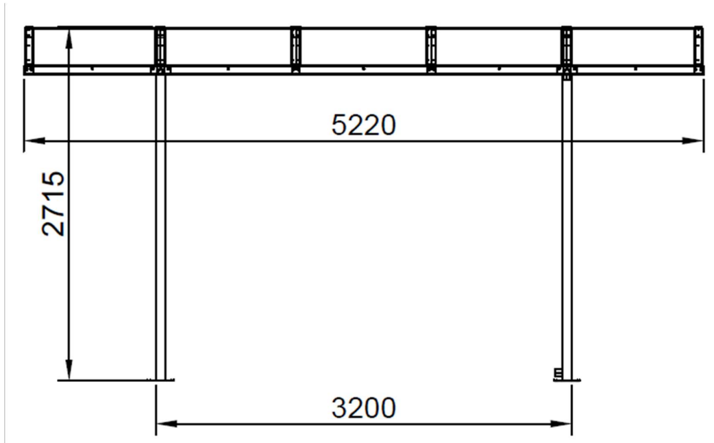
Mål tegning (set fra siden)
