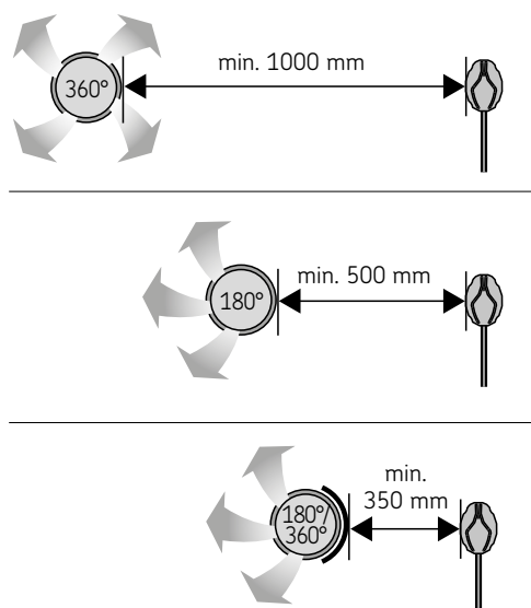
Рисунок 4.. Минимальное расстояние от температурного датчика до вентиляционной отдушины. Joonis 4. Ventilatsiooniva minimaalne kaugus andurist.
