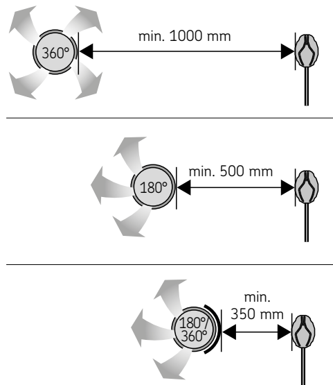
Figure 4. Minimum distance from the supply air vent to the temperature sensor. Abbildung 4. Mindestabstand des Fühlers zur Luftzufuhr.
