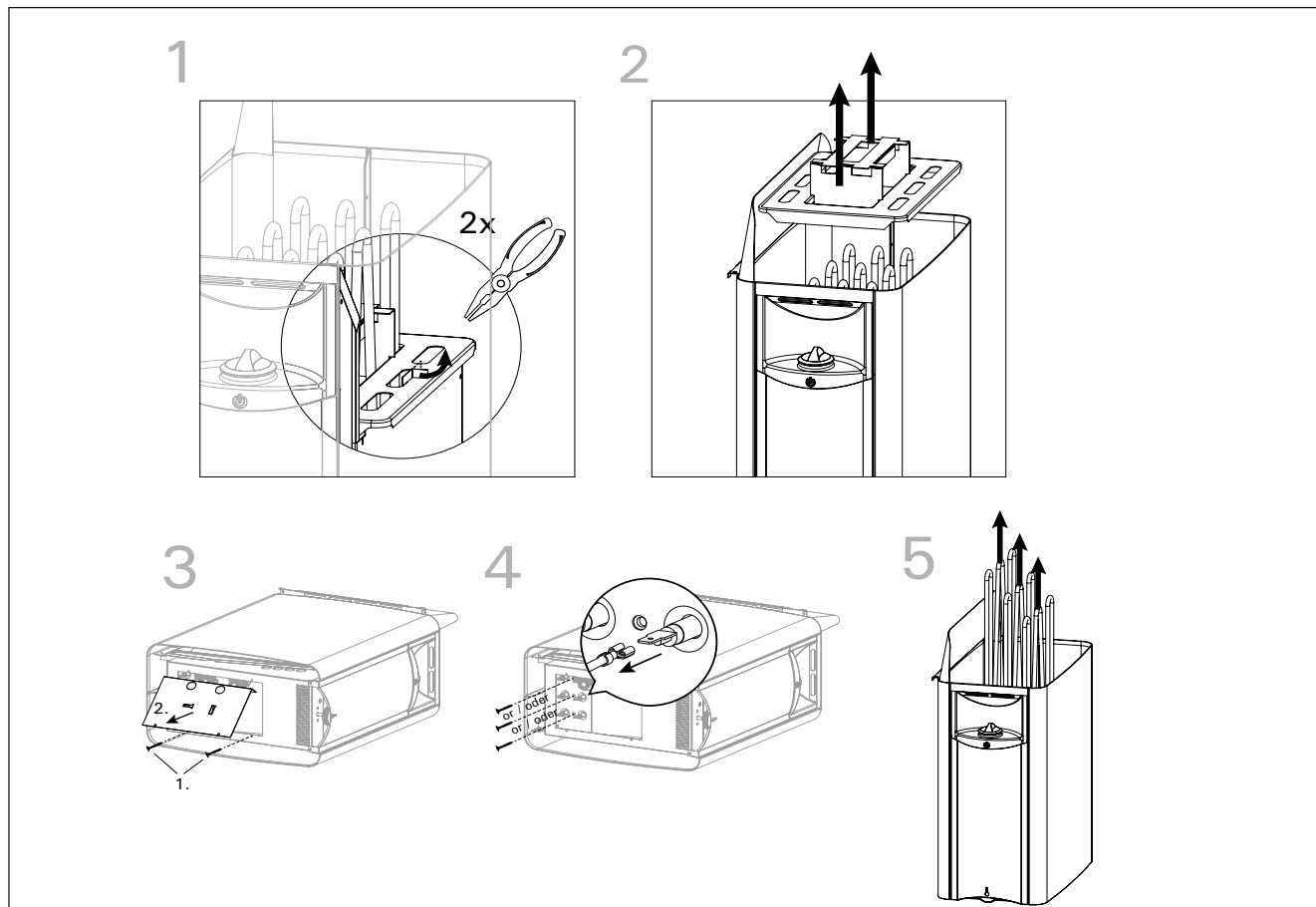
Figure 10. Replacing the Heating element Abbildung 10. Austausch der Heizstäbe
