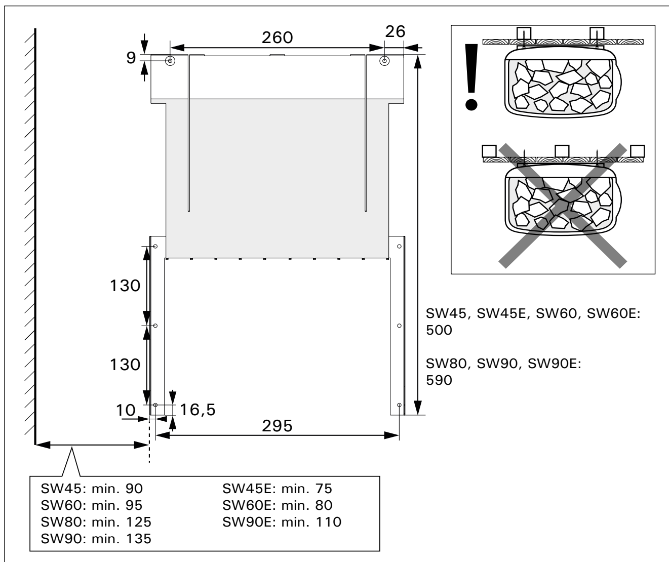
Рисунок 7. Настенный кронштейн, размеры в миллиметрах Joonis 7. Seinakinnitusraam, mõõdud millimeetrites
