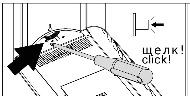
Рисунок 12. Восстановление рабочего состояния после срабатывания режима защиты от перегрева Joonis 12. Ülekuumenemiskaitse tagastamine
