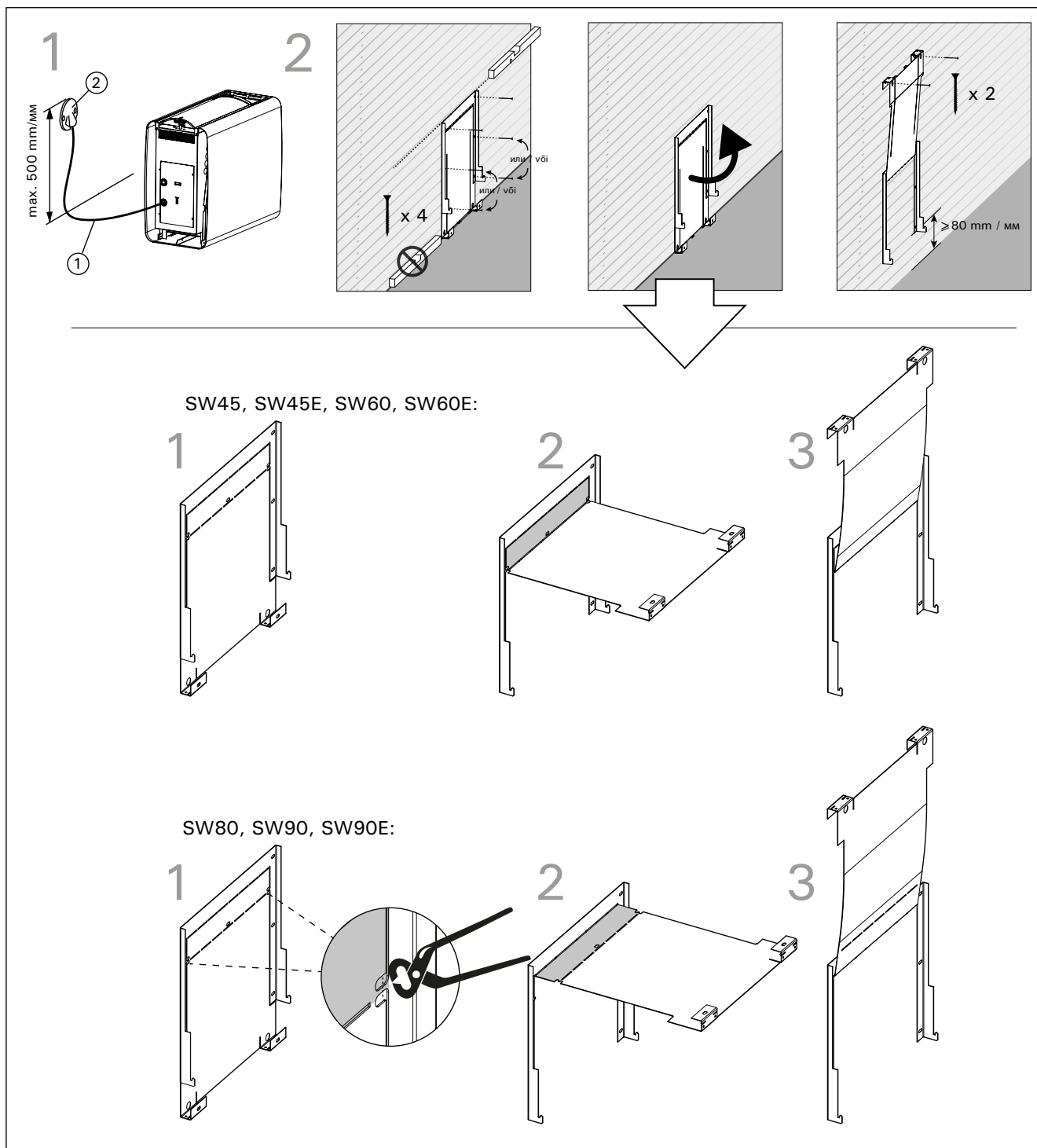
Рисунок 8. Крепление настенного кронштейна Joonis 8. Seinakinnitusraami paigaldamine
