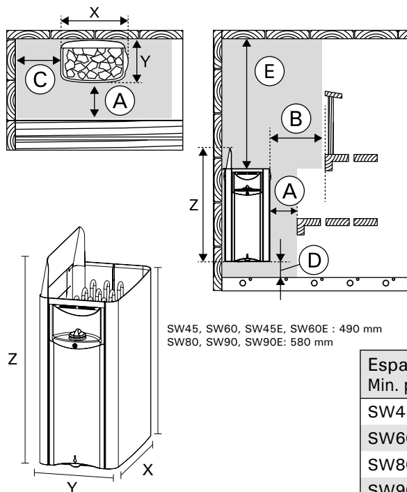
Figure 5. Distances de sécurité minimum (toutes les mesures sont indiquées en millimètres)
