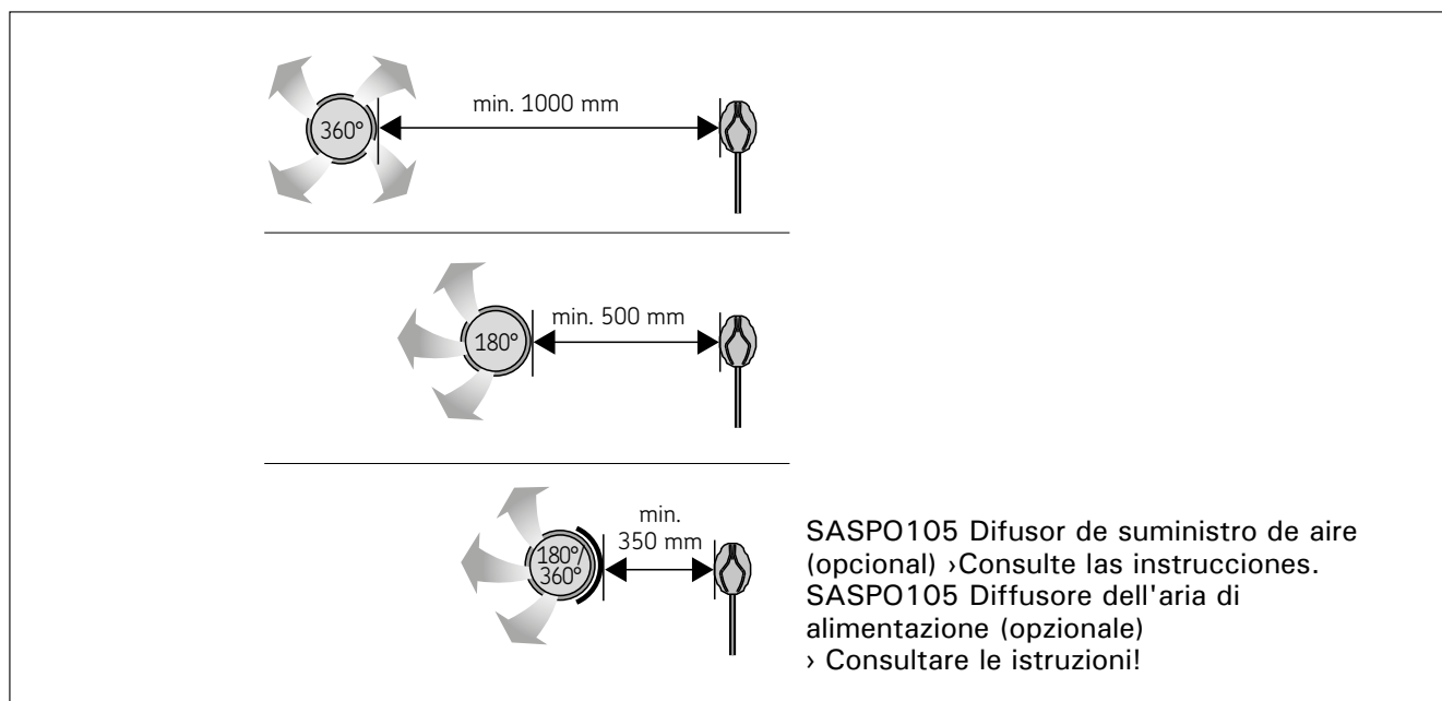
Figure 4. Distance minimale entre la bouche d'air et le capteur
