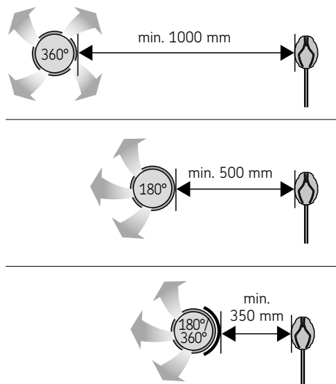
Kuva 4. Tuloilmaventtiilin vähimmäisetäisyys lämpötila-anturiin. Bild 4. Minimiavstånd mellan tilluftsventil och temperaturgivare.
