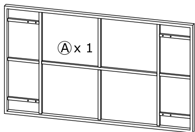
Top Table 1450x850x50 mm
