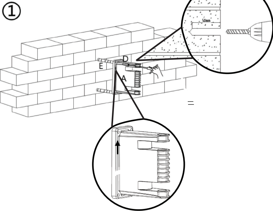
Assembly of the handle only with the arrow pointing up Montaż uchwyty wyłącznie strzałką skierowaną do góry
