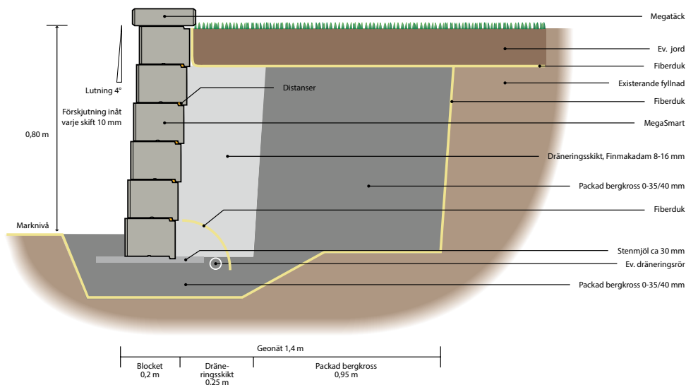
Bild 5. Sektionsritning lutande stödmur utan geonät, upp till 0,8 m.
