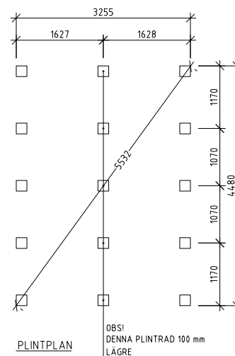
Plantegning
