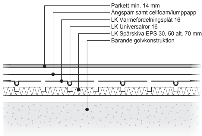
LK EPS 30/50/70 förlagt flytande på bärande golv. Ytskikt parkett.
