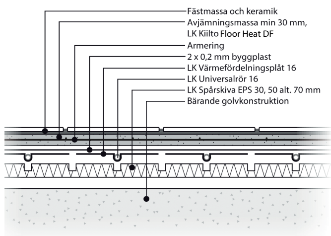
LK EPS 30/50/70 förlagt på bärande golv i torrt utrymme med LK Kiilto Floor Heat DF. Keramiskt ytskikt.
