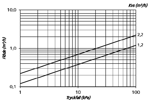
KAPACITETSDIAGRAM
